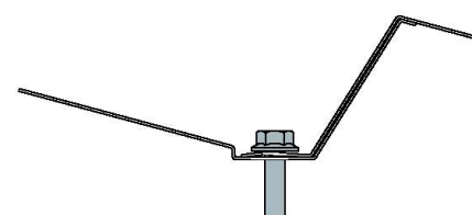
DETALLE SOLAPE Y SUJECIÓN
